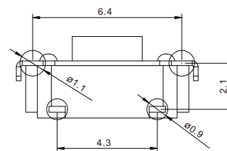
安装图 instructions
